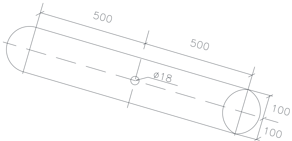
Figura 103 - Morto
