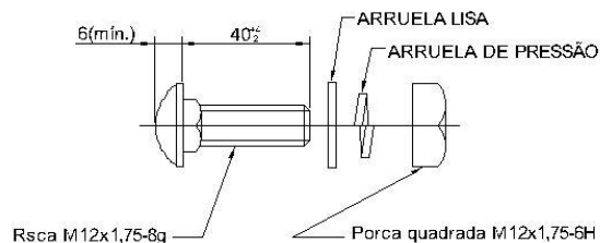
Figura 134 - Suporte T
