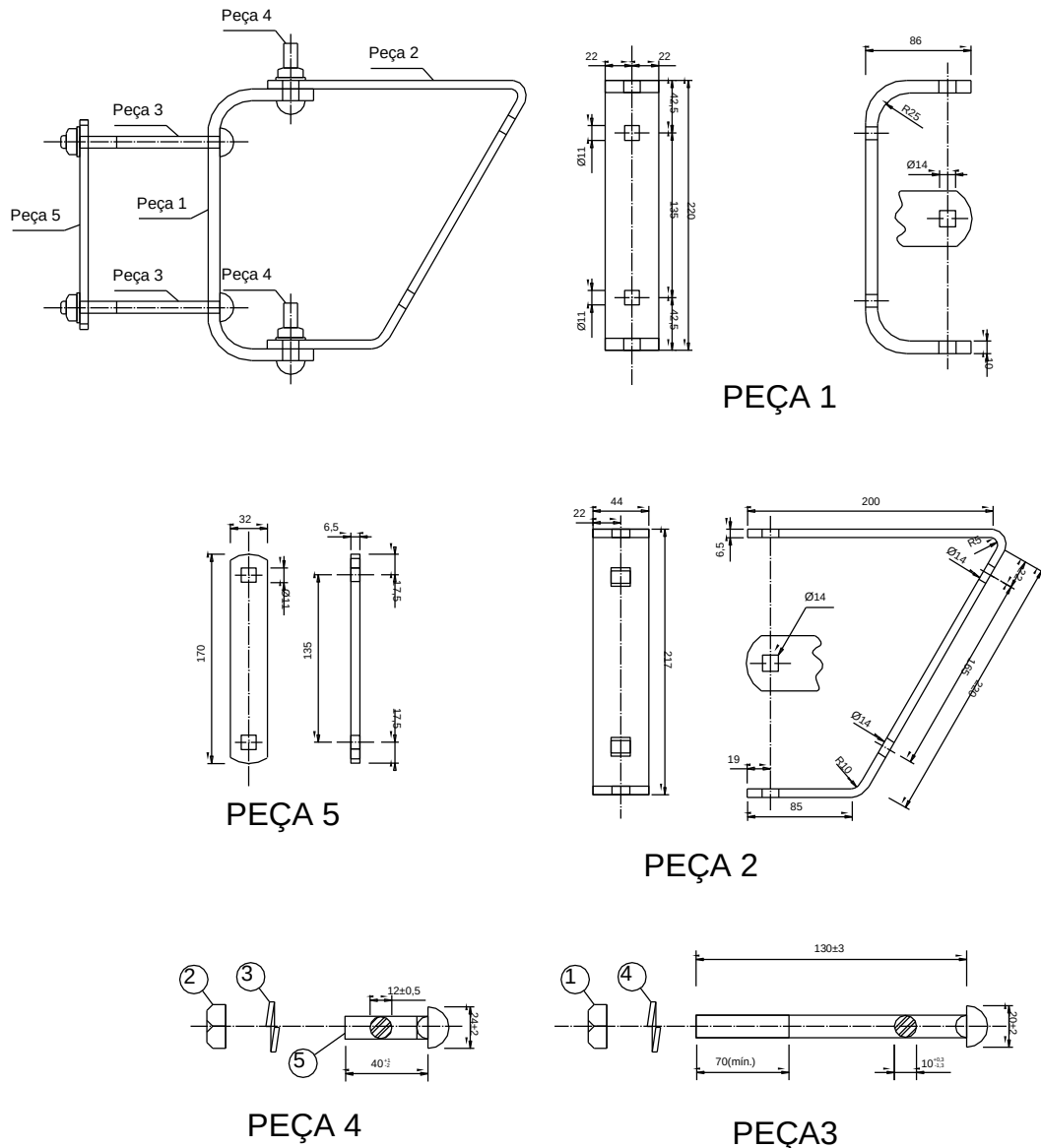
Figura 130 - Suporte para fixação inclinada de chave faca
