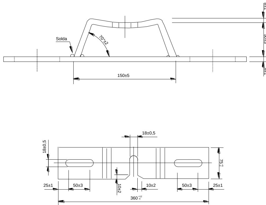
Figura 131 - Suporte para transformador - Poste de madeira
