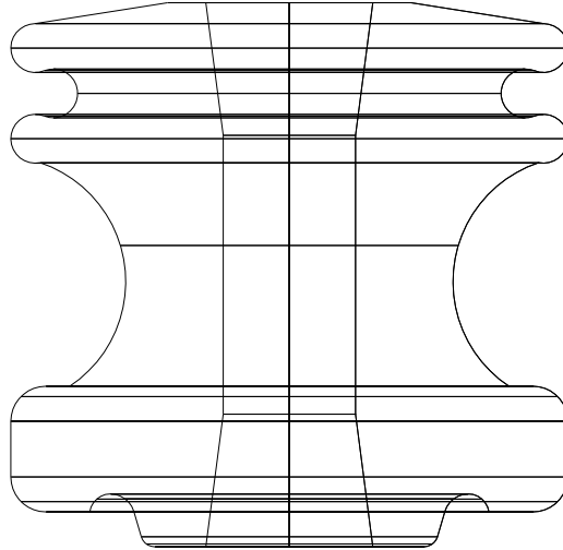
Figura 90 - Isolador tipo roldana
