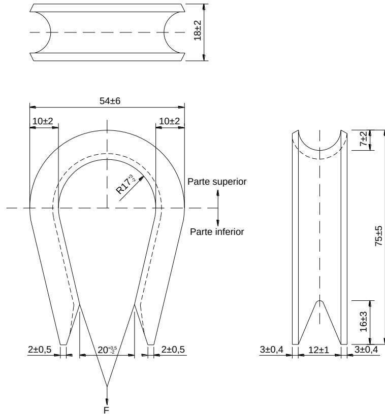
Figura 121 - Sapatilha
