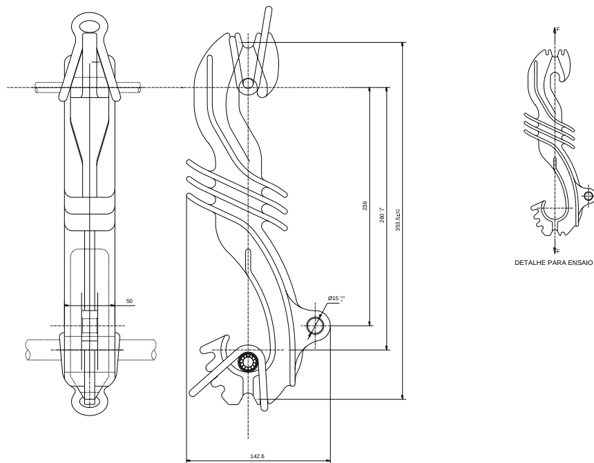
Figura 71 - Espaçador monofásico
