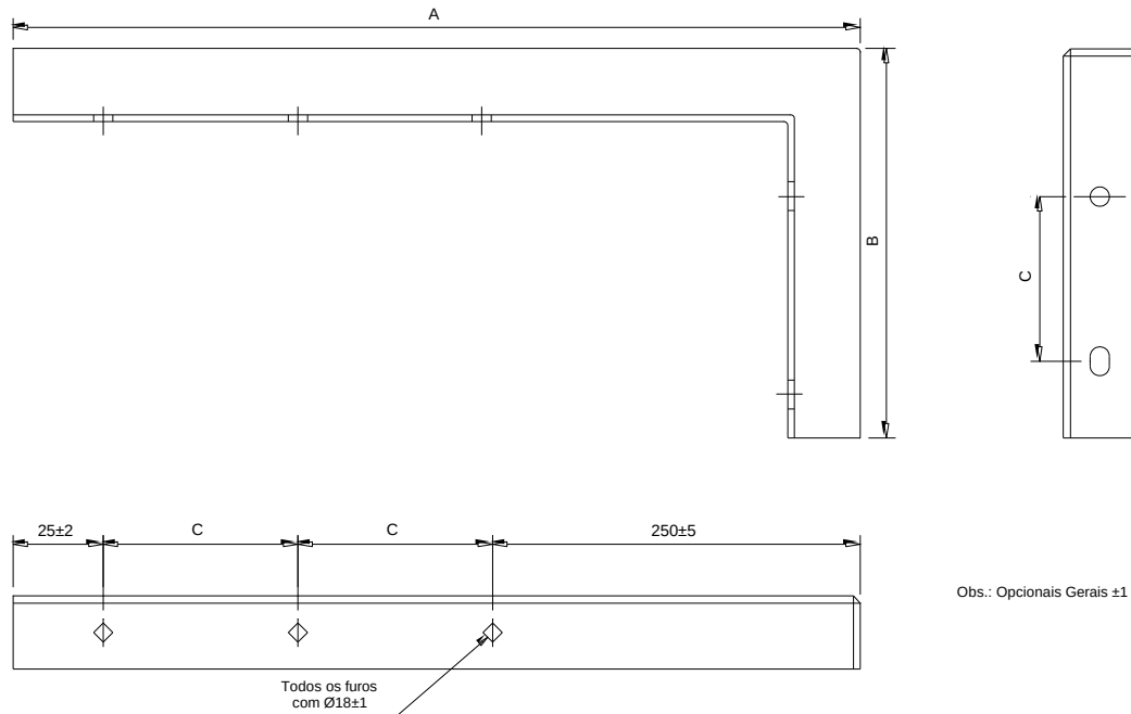
Figura 127 - Suporte horizontal
