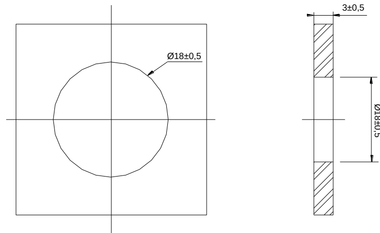
Figura 14 - Arruela quadrada
