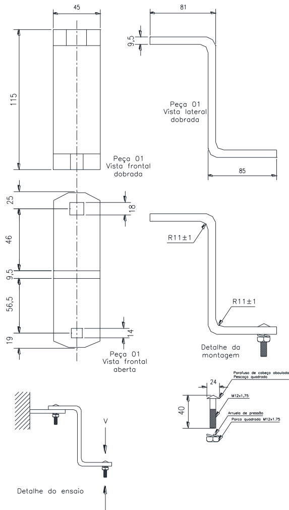
Figura 136 - Suporte Z
