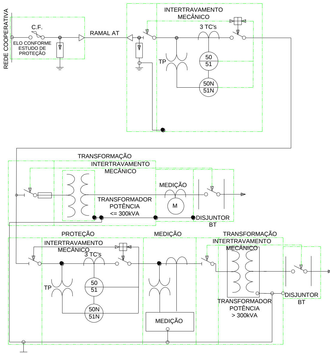
Figura 42 – Esquema básico de Subestação Compartilhada
