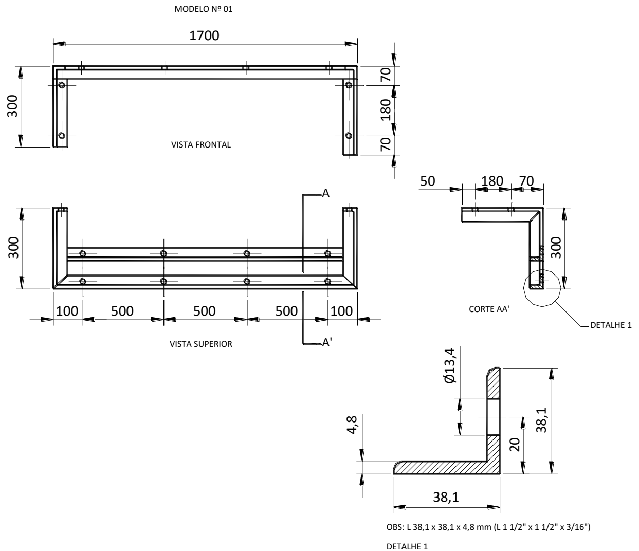
Figura 34 - Suporte para mufas
