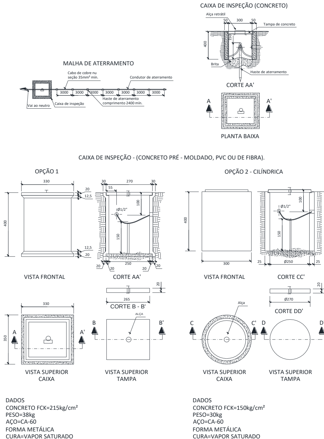
Figura 40 - Aterramento
